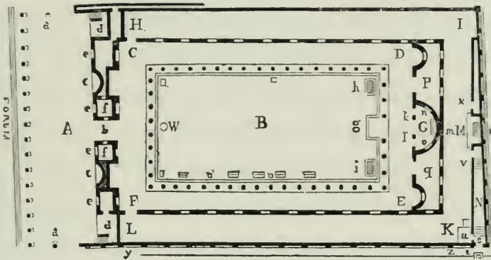
Plan de l'édifice d'Eumachia.
