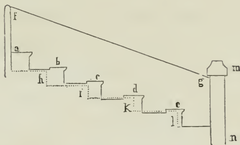
Coupe de la première Cavea.
