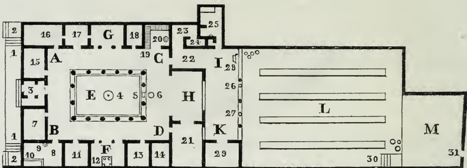
Plan de la Maison d'Epidius Rufus.
