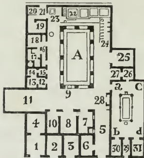
Plan de la Fullonica.
