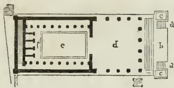
Plan du Temple de Jupiter.
